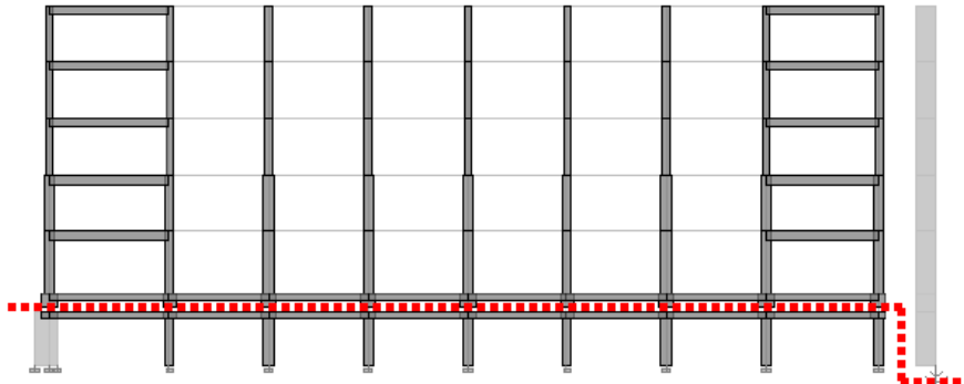
Figura 1-1: Esquema del sistema de aislamiento: nivel de aislamiento en línea segmentada.
