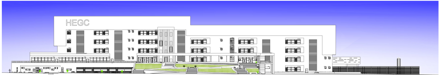
ELEVACIÓN NORTE
